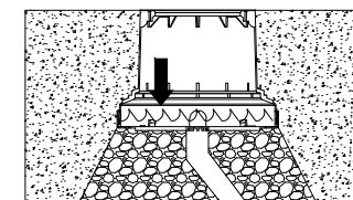
Drenaggio corretto - Correct drainage
